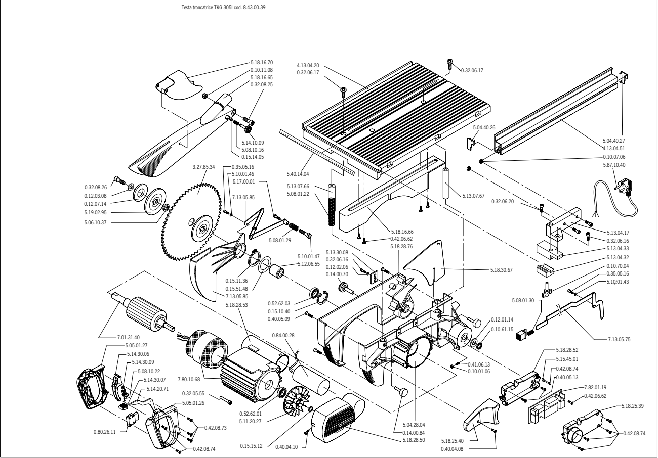
Testa troncatrice TKG 305i cod. 8.43.00.39
