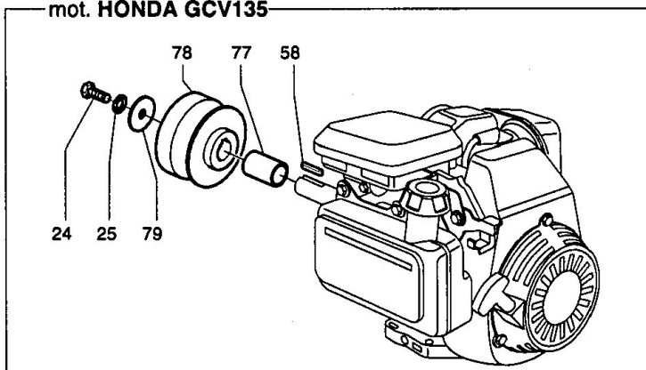
mot. HONDA GCV135
